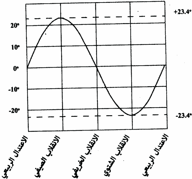
الشكل (85): ميل الشمس خلال العام بافتراض مدار دائري تام.
